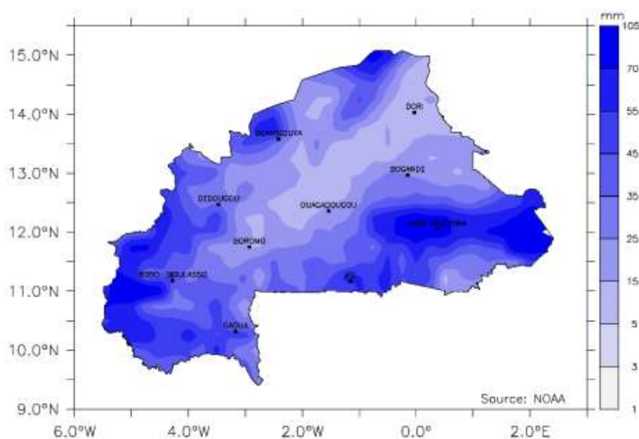
Figure 13 : Cumul pluviométrique allant de la période du 04 au 10 juillet 2015
