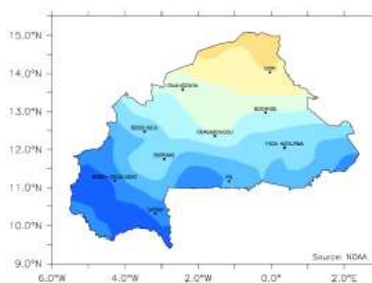
Figure 14a : Températures minimales pour la juillet 2015
