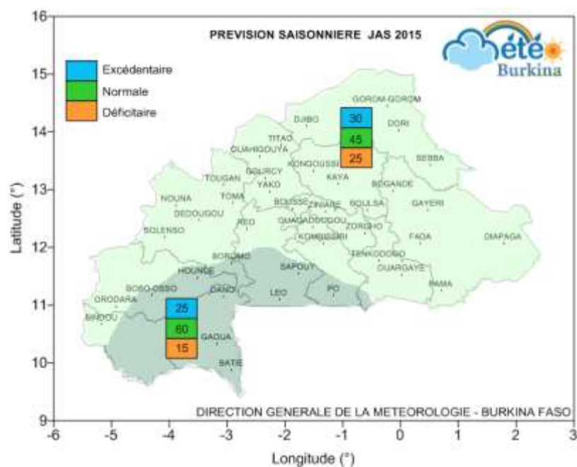
Figure 15 : Prévion saisonnière du cumul pluviométrique JAS 2015
