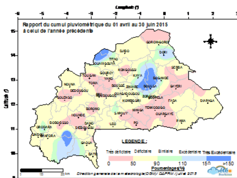
Figure 5 : Rapport du cumul pluviométrique du 01 avril au 30 juin 2015 et celui de l'année précédente.
