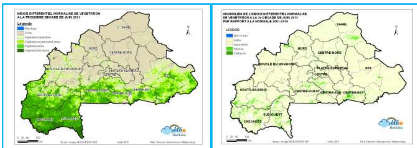
Fig.12 : Anomalies des différences d'images d'indices de végétation entre la troisième décennie de juin 2015 et la moyenne 2001-2010
