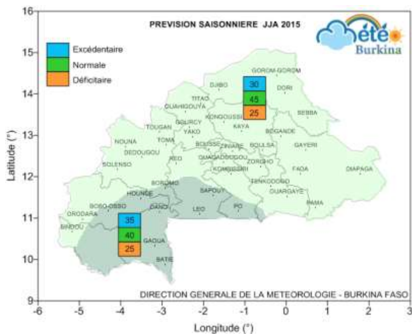
Figure 14 : Prévion saisonnière du cumul pluviométrique JJA 2015
