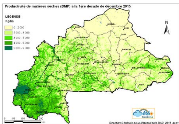
Figure Oc : Productivité de matière sèche à la première décade de décembre 2015
