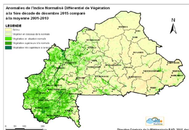
Figure Ob : différence des indices de végétation entre la 1 ère décade de décembre 2015 et la moyenne 2001-2010
