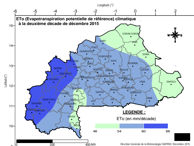
Figure m : Prévision climatologique de l'ETo à la deuxième décennie de décembre 2015
