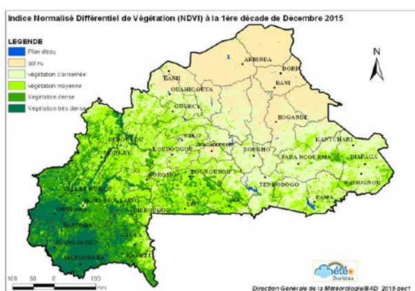
Figure Oa : niveau de couverture de la végétation à la première décade de décembre 2015
