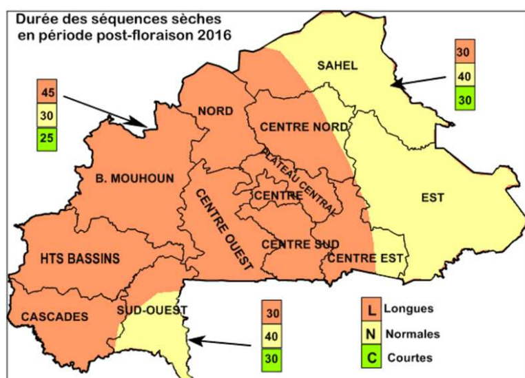
Figure 18 : Durées probables des séquences sèches en fin de saison des pluies
