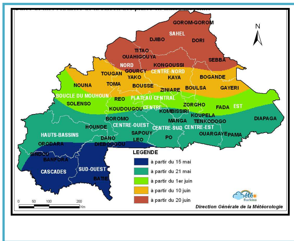
Figure 10 : dates de début climatologiques moyennes de la saison des pluies
