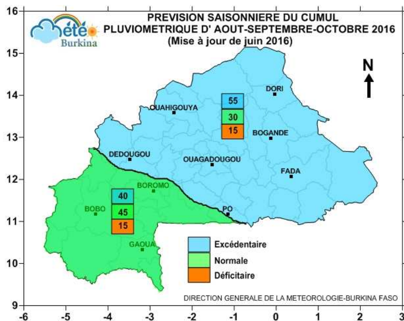
Figure 14 : Prévision saisonnière du cumul pluviométrique ASO 2016
