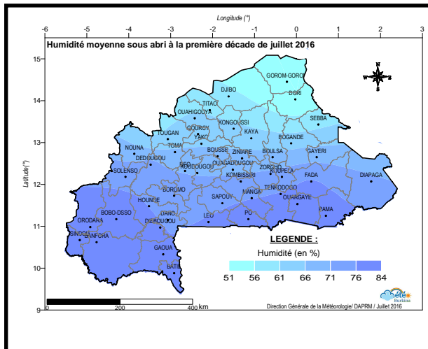
Fig. 8 : Evolution de l'humidité relative moyenne à la première décade de juillet 2016
