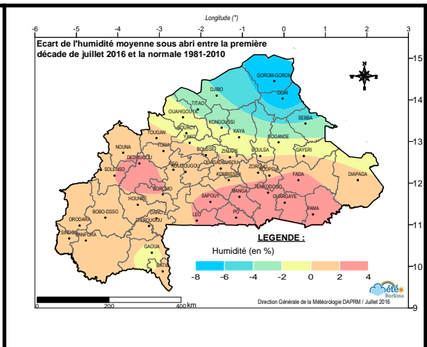
Fig. 9: Ecart de l'humidité moyenne entre la première décade de juillet 2016 et la moyenne (1981-2010)
