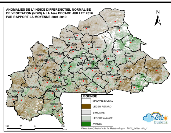
Fig.12 : NDVI à la 1 ère décennie de juillet 2016 comparé à la moyenne 2001-2010
