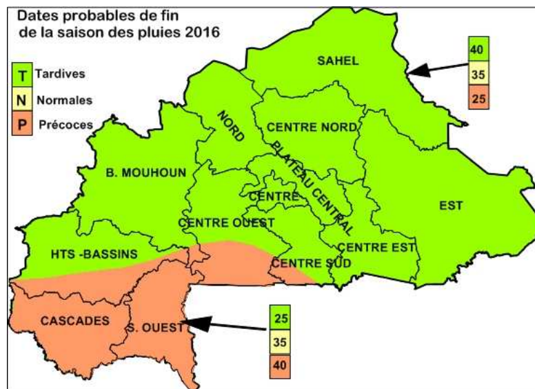
Figure 16 : Tendances probables des dates de fin de la saison des pluies
