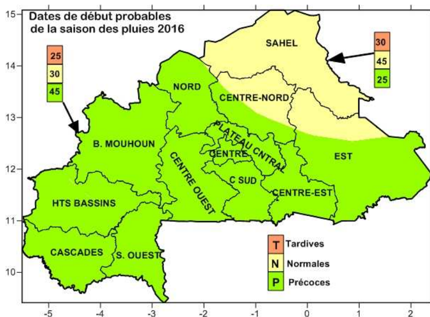
Figure 15: dates probables de début de la saison des pluies
