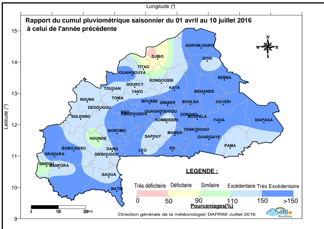
Figure 5 : Rapport du cumul pluviométrique du 1 er avril au 10 juillet 2016 et celui de l'année précédente.
