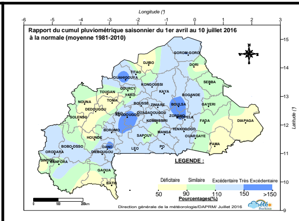
Figure 4 : Rapport du cumul pluviométrique du 1 er avril au 10 juillet 2016 et la normale 1981-2010
