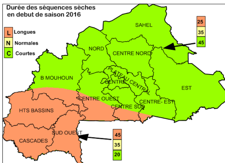
Figure 17 : Durées probables des séquences sèches en début de saison des pluies
