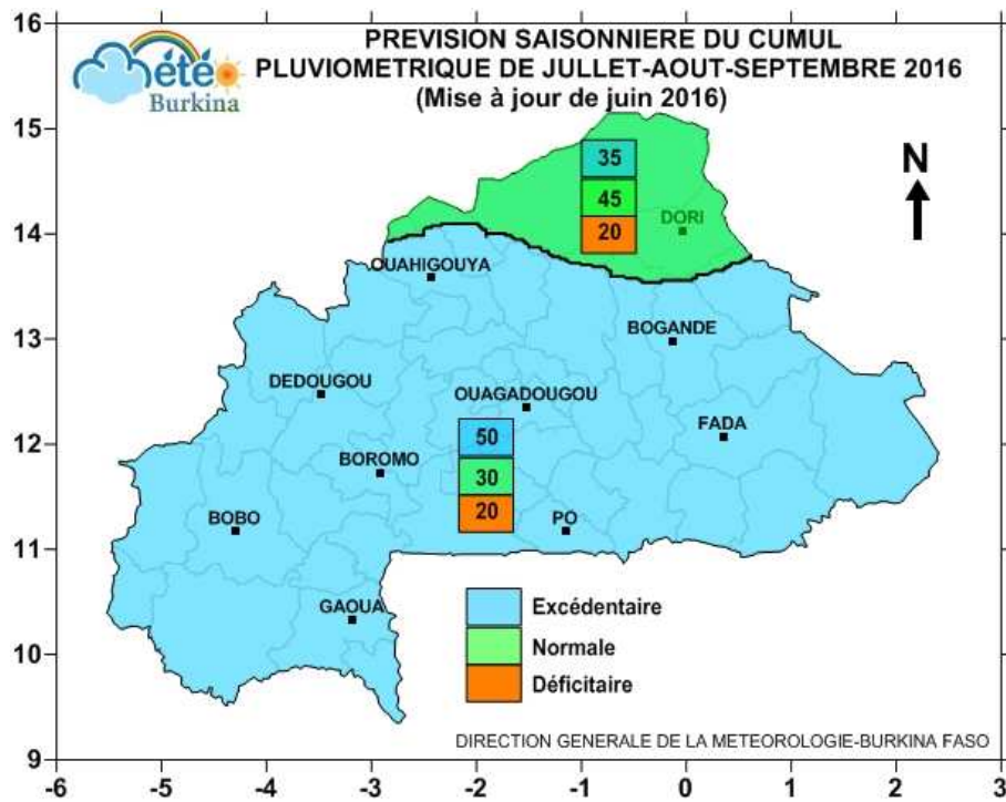
Figure 13 : Prévision saisonnière du cumul pluviométrique JAS 2016
