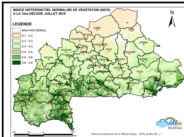
Fig.11 : NDVI à la 1 ère décennie de juillet 2016
