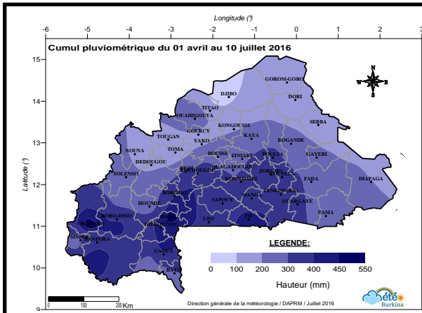
Figure 3 : Cumul pluviométrique saisonnier du 01 avril au 10 juillet 2016
