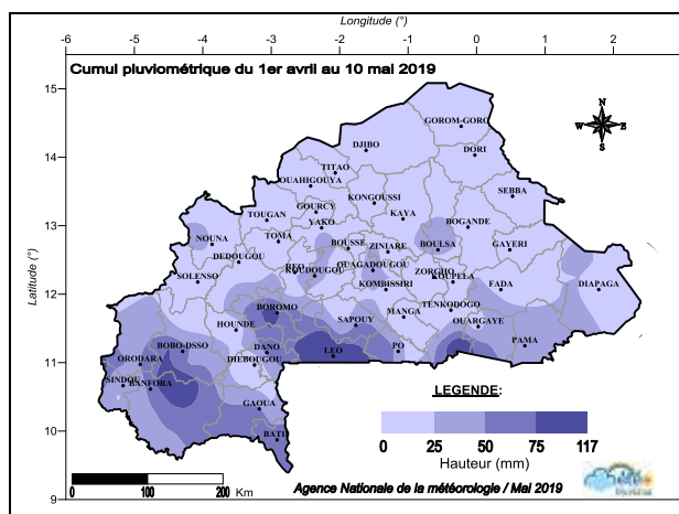
Figure 3 : Cumul pluviométrique saisonnier du 01 avril au 10 mai 2019
