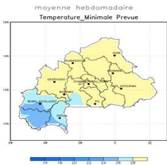
Figure 13 : NOAA températures minimales prévues du 11 au 18 mai 2019
