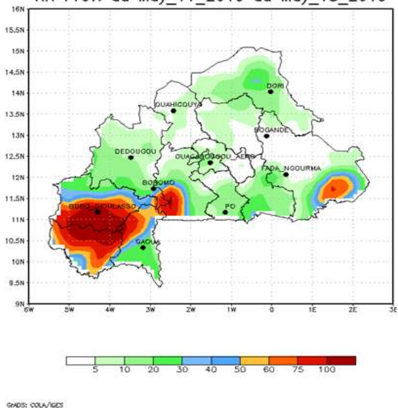
Figure 12 : NOAA : cumul pluviométrique attendu du 11 au 18 mai 2019
