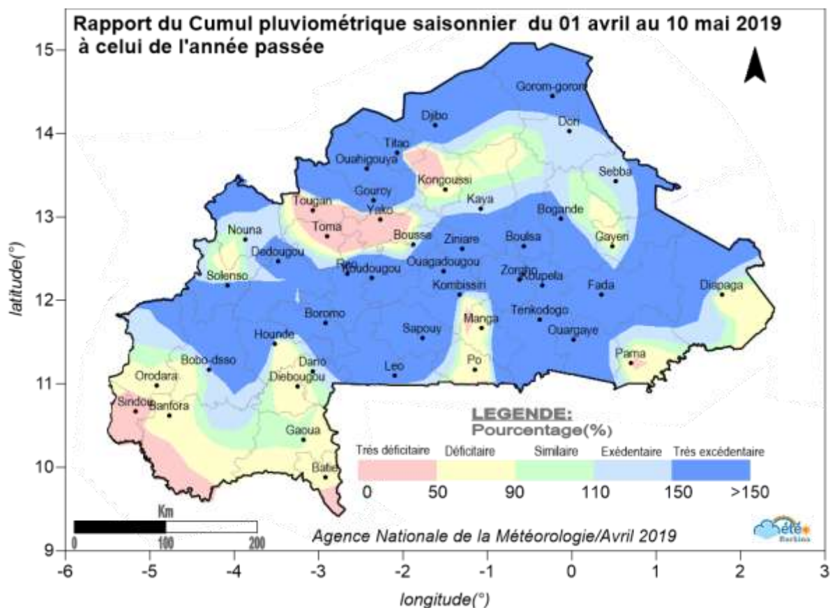
Figure 5 : Rapport du cumul pluviométrique du 1 er avril au 10 mai 2019 à celui de l'année précédente
