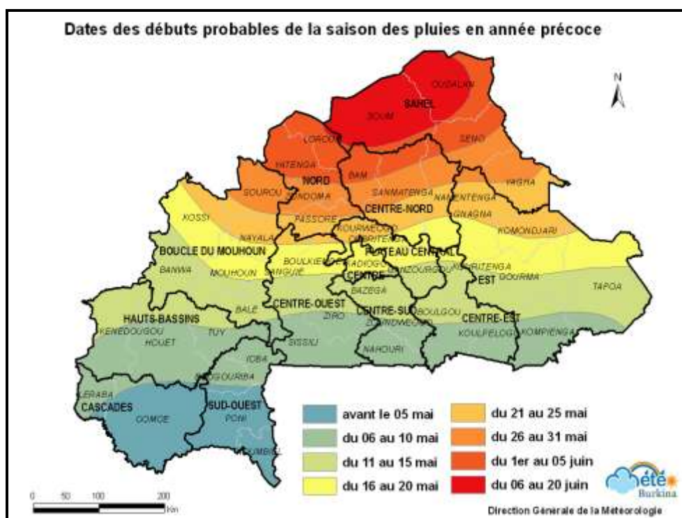
Fig. 10 : dates de début précoce de la saison des pluies (1 an sur 5)
