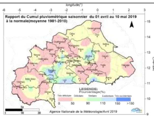
Figure 4 : Rapport du cumul pluviométrique du 1er avril au 10 mai 2019 à la normale 1981-2010
