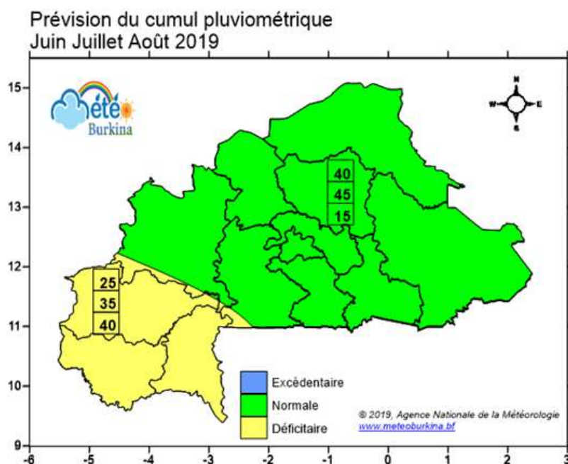
Figure 15 : Prévision saisonnière du cumul pluviométrique JJA 2019
