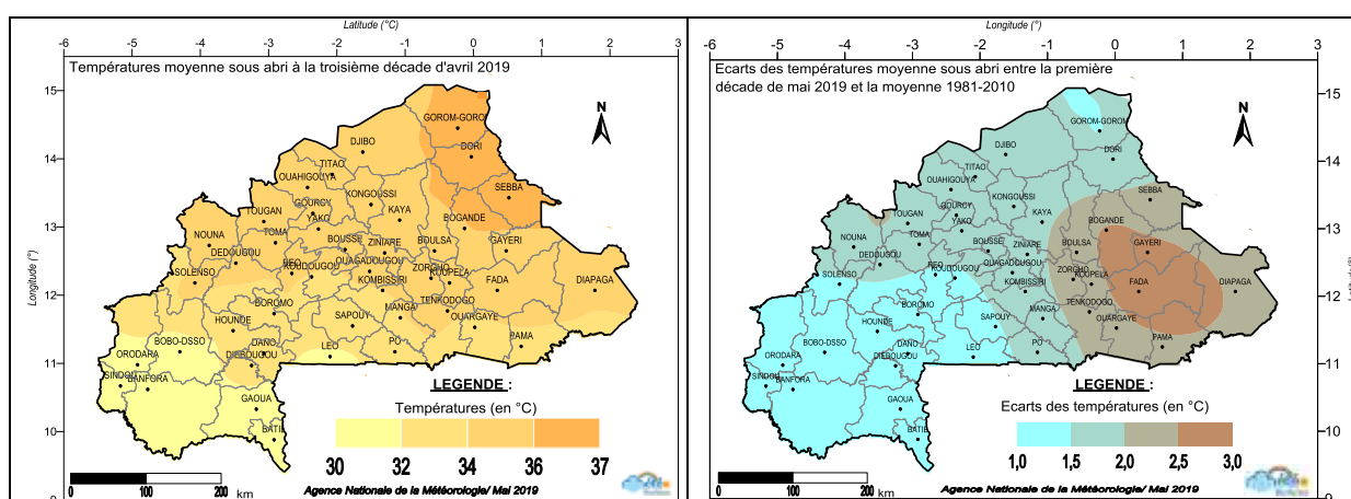
Figure 6 : Températures moyennes sous abri à la première décade de mai 2019.
