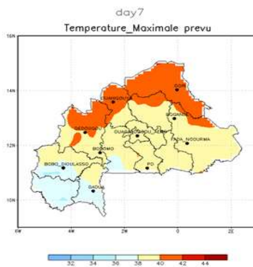
Figure 14 : NOAA températures maximales prévues du 11 au 18 mai 2019
