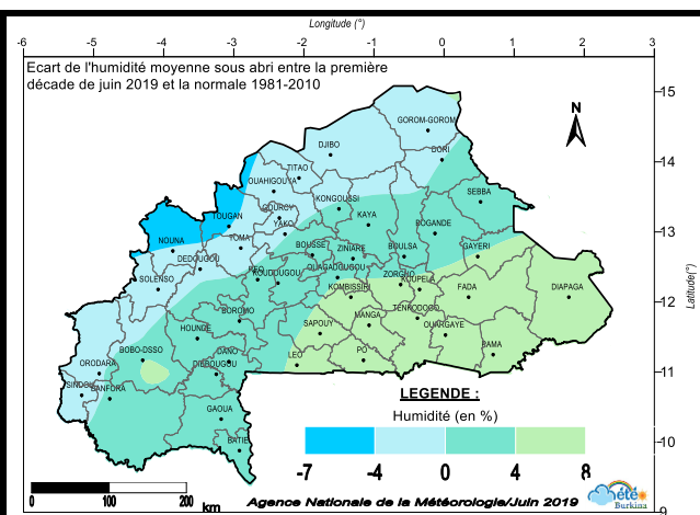
Figure 9 : Ecart de l’humidité relative moyenne entre la première décade de juin 2019 et la moyenne (1981-2010).
