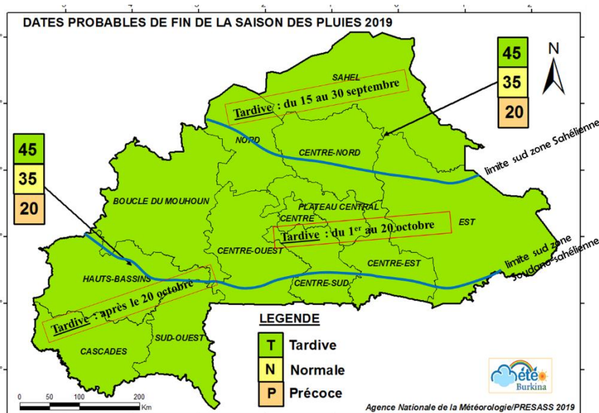
Figure 20 : Tendances probables des dates de fin de la saison des pluies 2019
