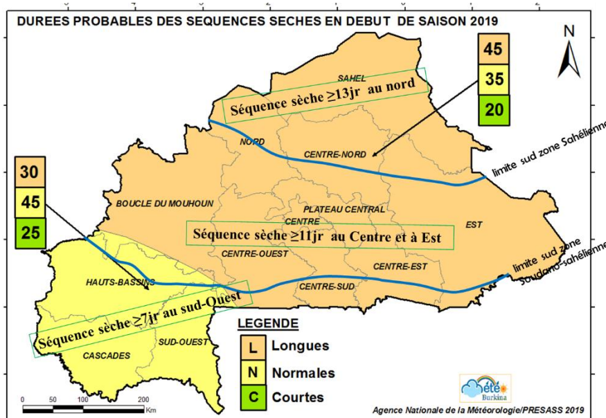
Figure 18 : Durées probables des séquences sèches en début de saison des pluies 2019
