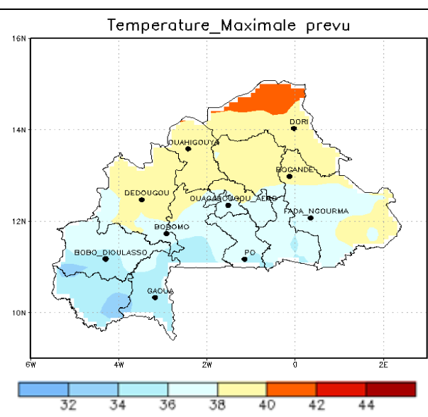
Figure 14 : NOAA températures maximales prévues du 12 au 18 juin 2019
