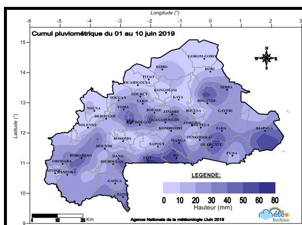
Figure 1 : Cumul pluviométrique à la première décade de juin 2019.
