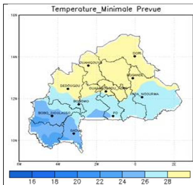
Figure 13 : NOAA températures minimales prévues du 12 au 18 juin 2019
