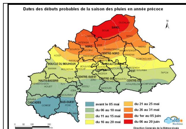
Fig. 10a : dates de début précoce de la saison des pluies (1 an sur 5)
