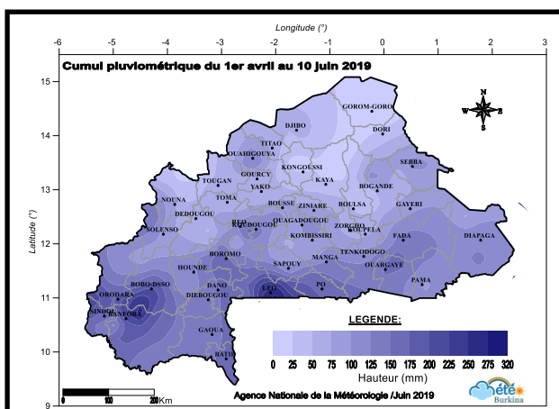
Figure 3 : Cumul pluviométrique saisonnier du 1 er avril au 10 juin 2019
