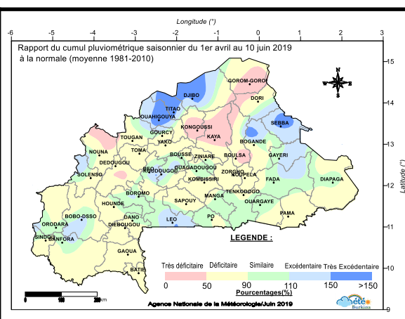
Figure 4 : Rapport du cumul pluviométrique du 1 er avril au 10 juin 2019 à la normale 1981-2010
