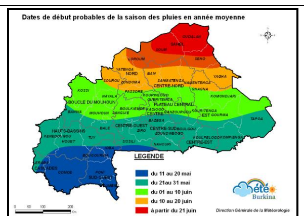
Fig. 10b : dates de début moyenne de la saison des pluies (1 an sur 2)
