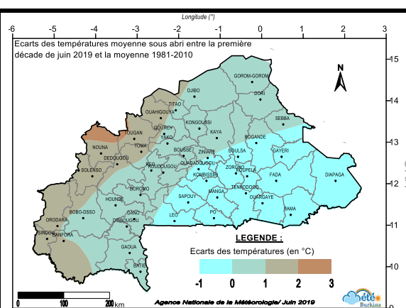
Figure 7 : Ecart des températures moyennes entre la première décade de juin 2019 et la moyenne (1981-2010).
