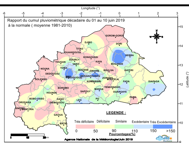
Figure 2 : Rapport du cumul pluviométrique à la première décade de juin 2019 et la normale 1981-2010.
