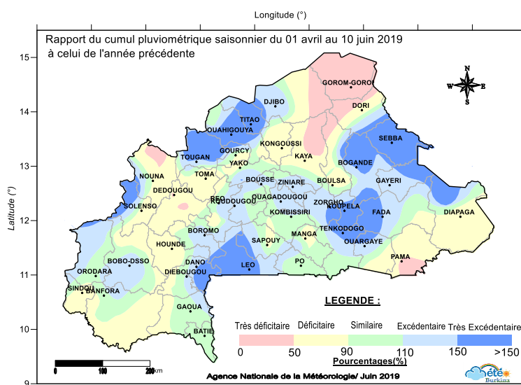
Figure 5 : Rapport du cumul pluviométrique du 1 er avril au 10 juin 2019 à celui de l'année précédente.
