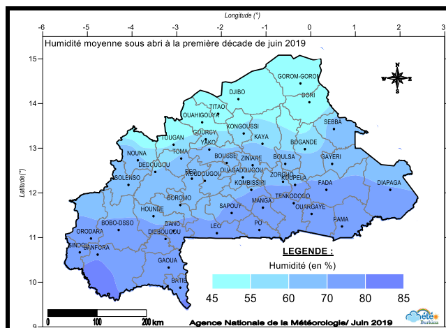
Figure 8 : Evolution de l’humidité relative moyenne à la première décade de juin 2019.
