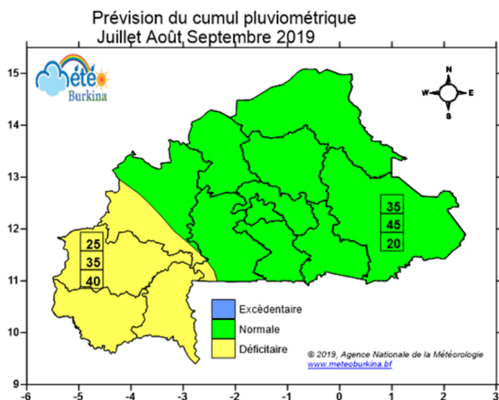
Figure 16 : Prévision saisonnière du cumul pluviométrique JAS 2019
