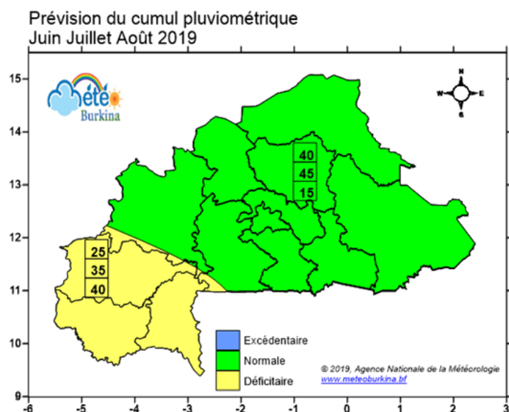
Figure 15 : Prévision saisonnière du cumul pluviométrique JJA 2019
