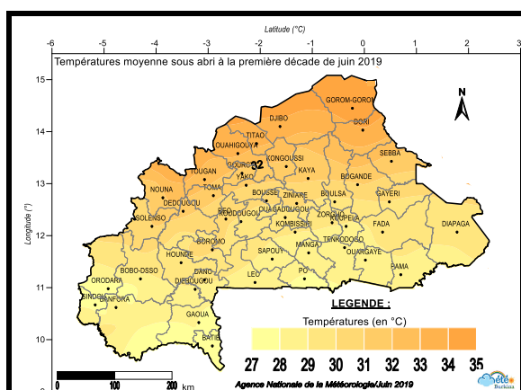
Figure 6 : Températures moyennes sous abri à la première décade de juin 2019.
