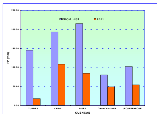
Gráfico 1 . Histograma de precipitación media - cuenca de la zona norte / vertiente del océano Pacífico
