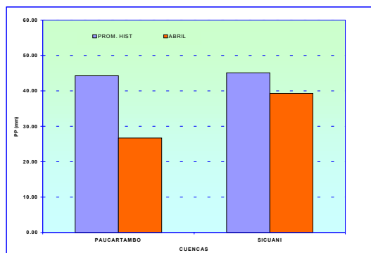
Gráfico 30. Histograma de precipitación - cuenca del río Vilcanota
