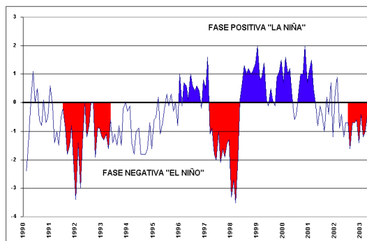
Figura 5. Índice de Radiación de Onda Larga
