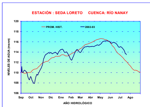
Gráfico 21. Limnigrama de niveles diarios del río Nanay
