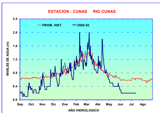
Gráfico 27. Limnigrama de niveles diarios del río Cunas
