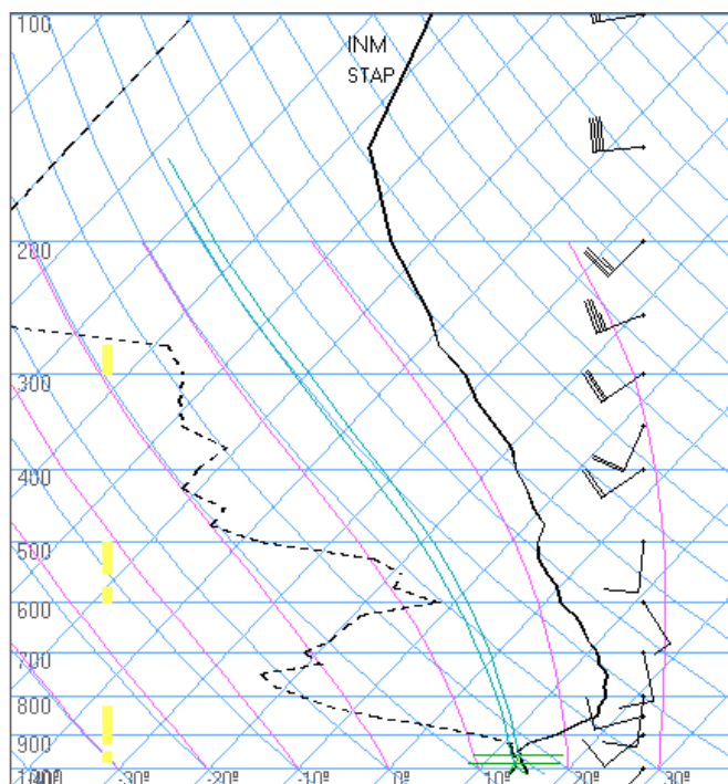
Figura 6. Radiosondaje mensual promedio - julio 2003 (Aeropuerto Internacional Jorge Chávez)
