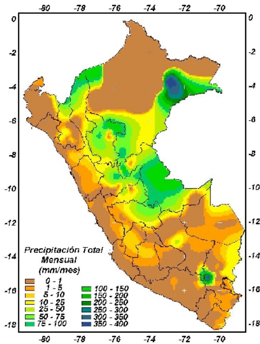
MAPA 5: Comportamiento mensual de la precipitación (mm/mes)
