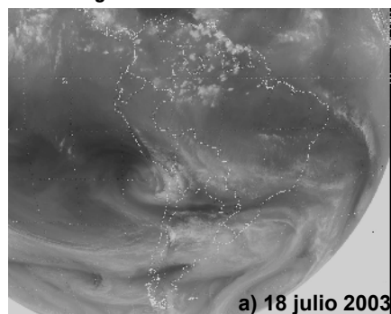
Figura 6. Imágenes satelitales de la ZCIT.
