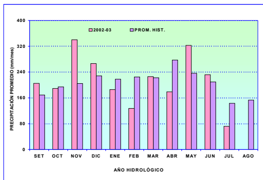
Gráfico 19. Histograma de precipitación regional en la selva norte
