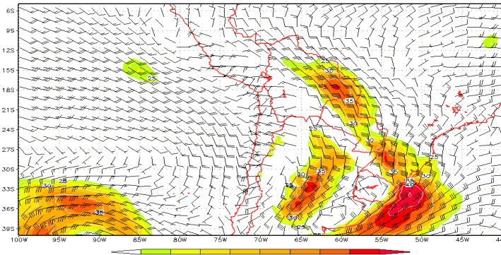
Figura 13. Isotacas e Isógonas (Kts), en el nivel de 850 hPa, con áreas sombreadas mayores a los 24 Kts (LLJ/SJ).
