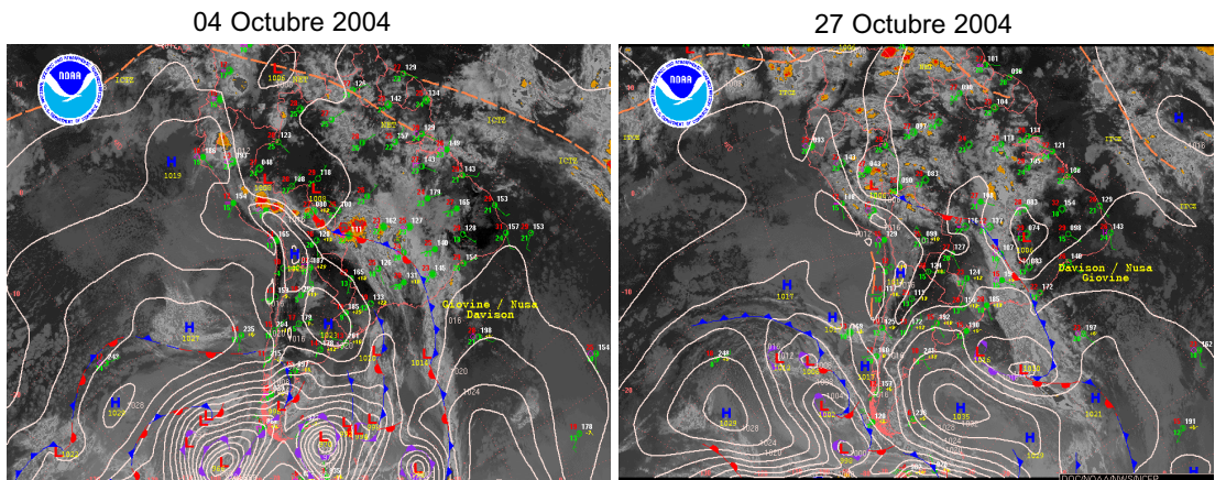
Figura 10. Imágenes satelitales y análisis sinóptico
